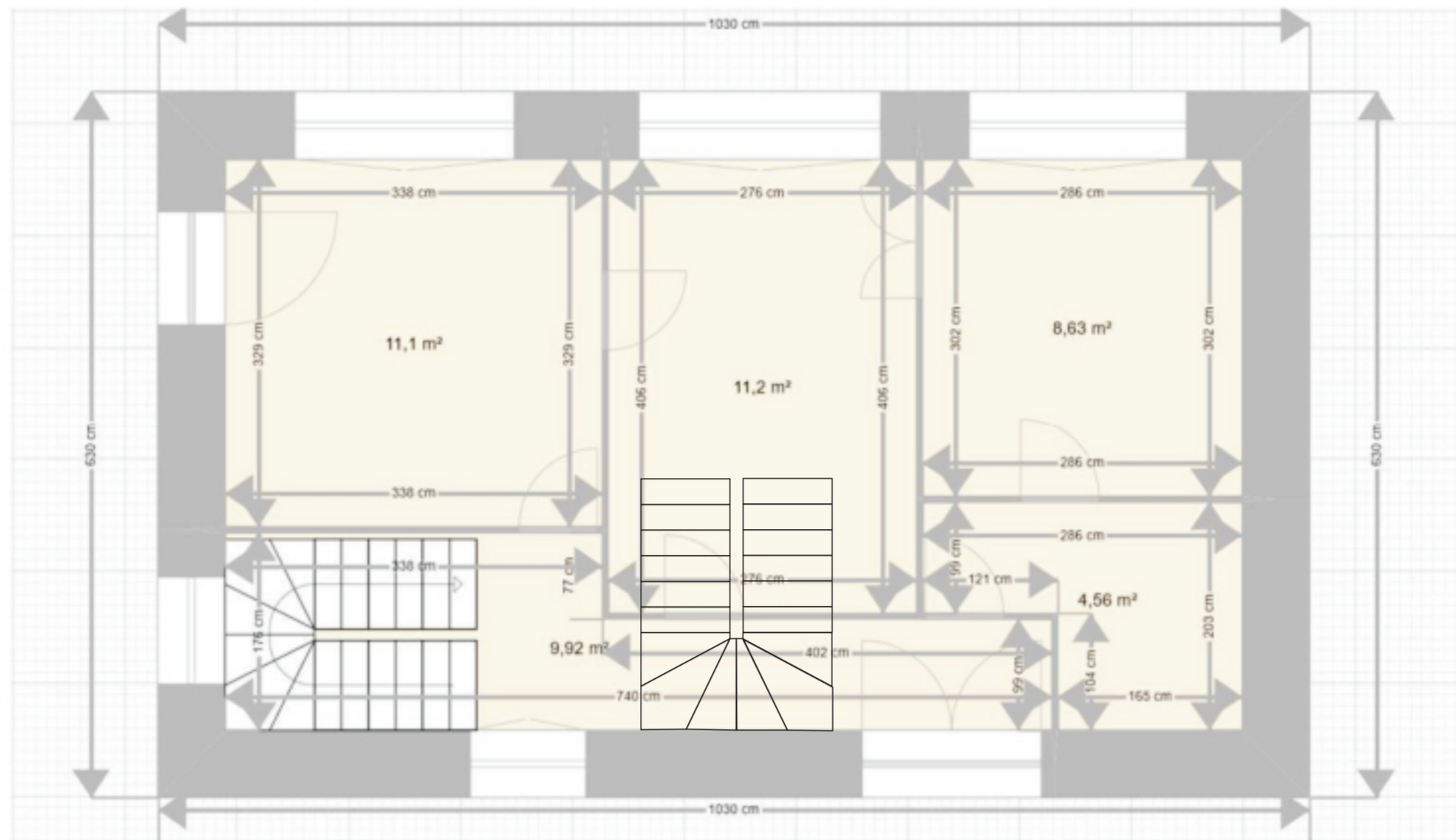
Plan du niveau 0
