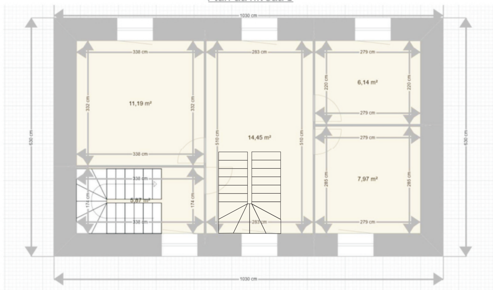
Plan du niveau 2
